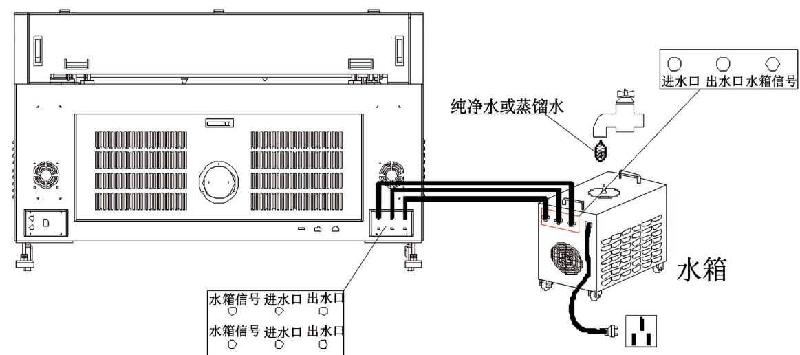
图 4-2 水箱连接
