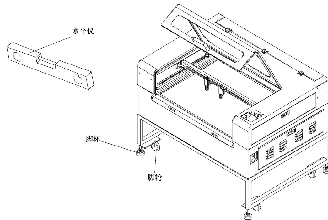
图 4-1 校水平
